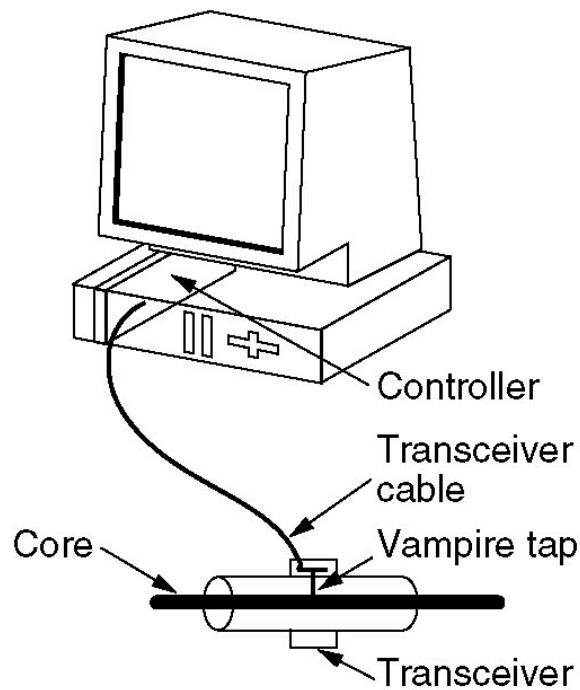
10Base5
